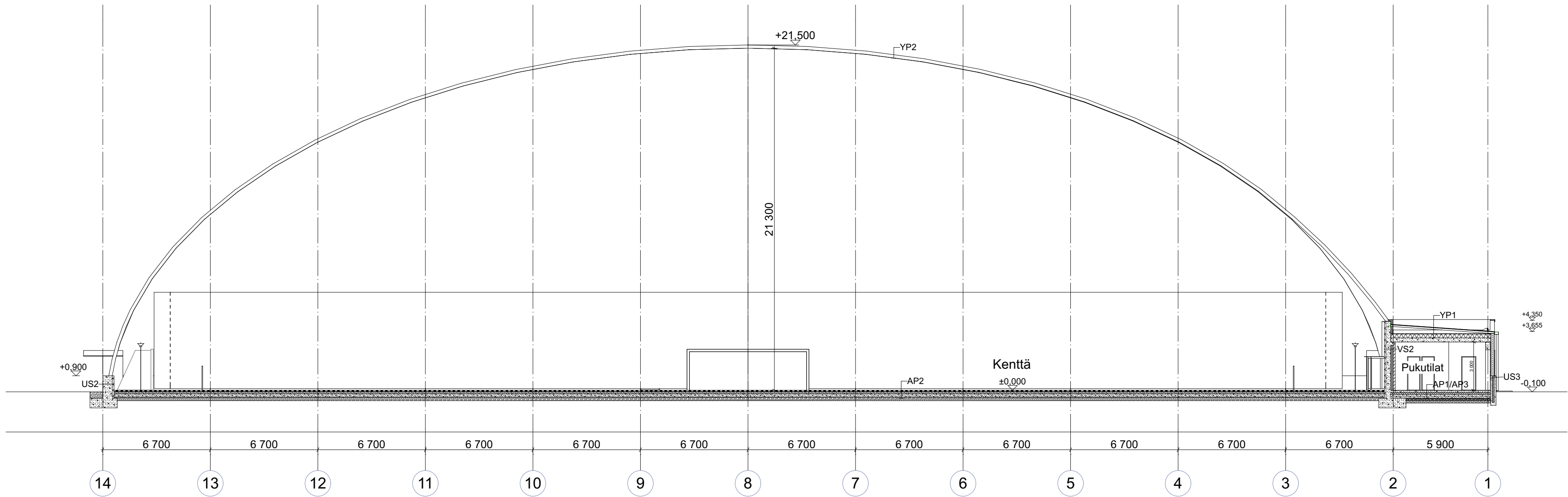
LEIKKAUS 1.
